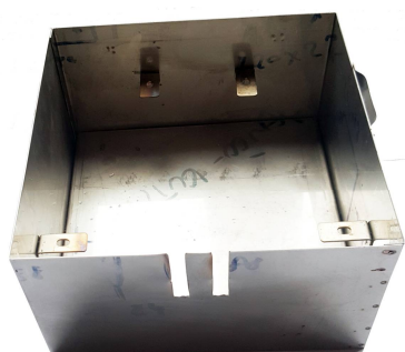
Kučište od inoxa dimenzija 200mm x 200mm x 100mm
